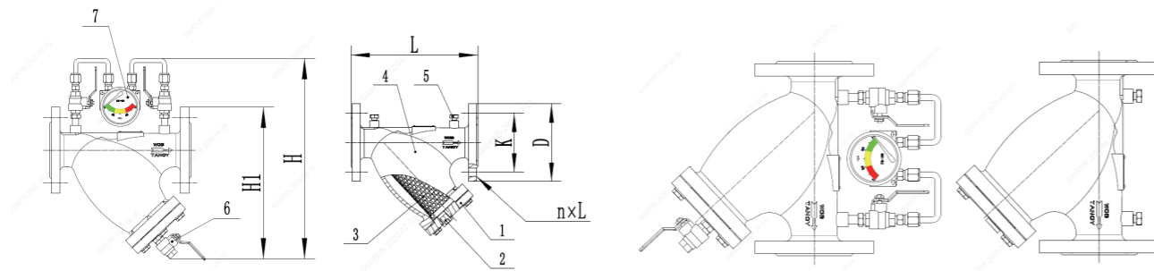
图 1 水平安装
