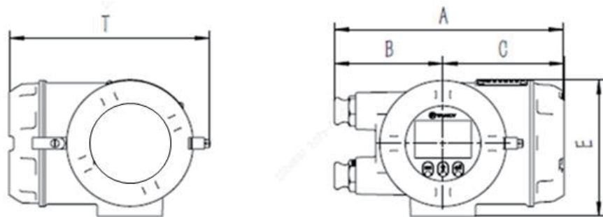
图 4 一体型变送器
