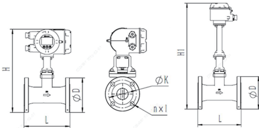
变送器一体型
