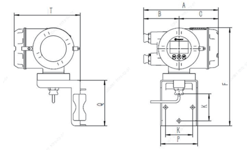
图 5 分体型变送器
