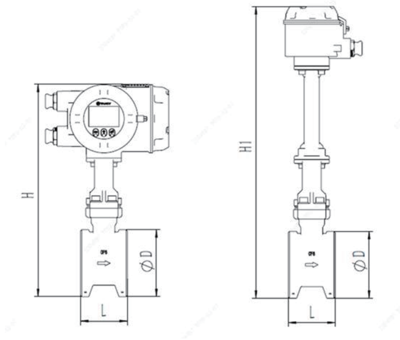
变送器一体型 图 3 夹持式外形尺寸图 变送器分体型
