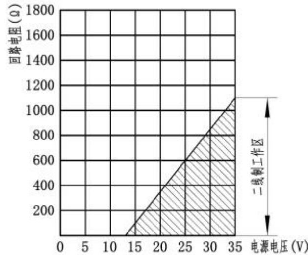
图 13 电源电压与回路电阻关系图
