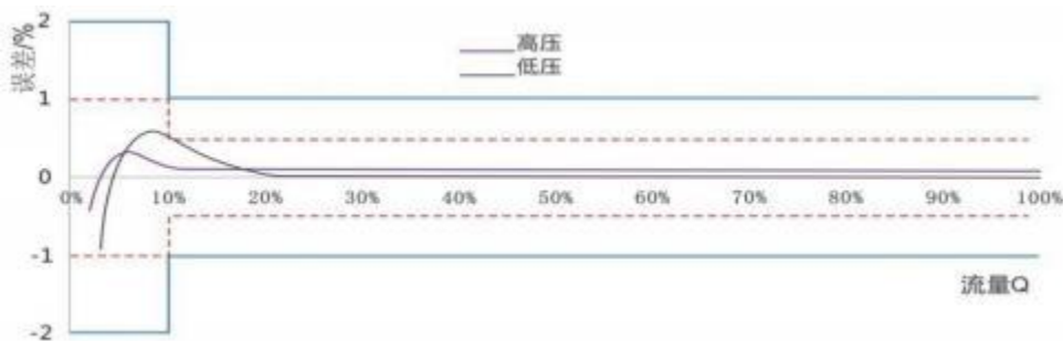
图 3 典型误差曲线图
