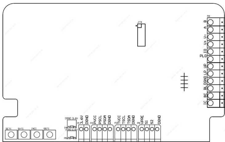
图 7 接线图
