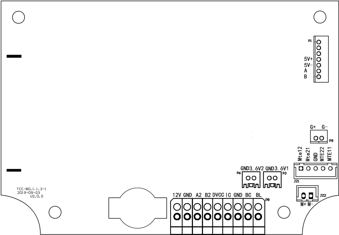
图 27-1 TCC-L 内部系统接线
