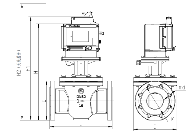
图 2-3 TCC-H 外型尺寸图
