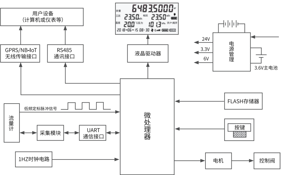
图 1 控制器原理框图
