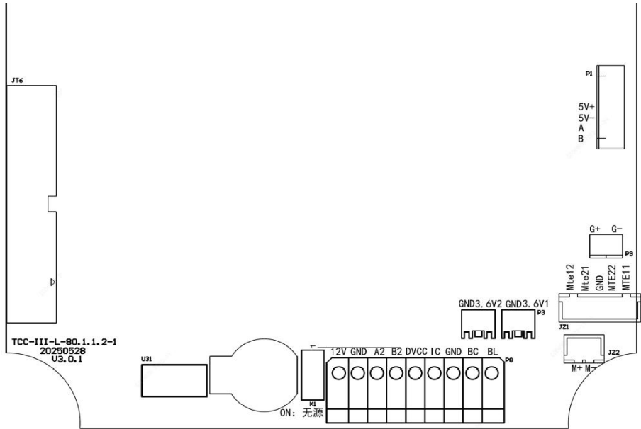
图 10-1 TCS-L, M (DN20~100) 内部系统接线
