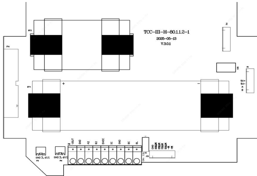
图 10-2 TCS-H、M (DN150~200) 内部系统接线
