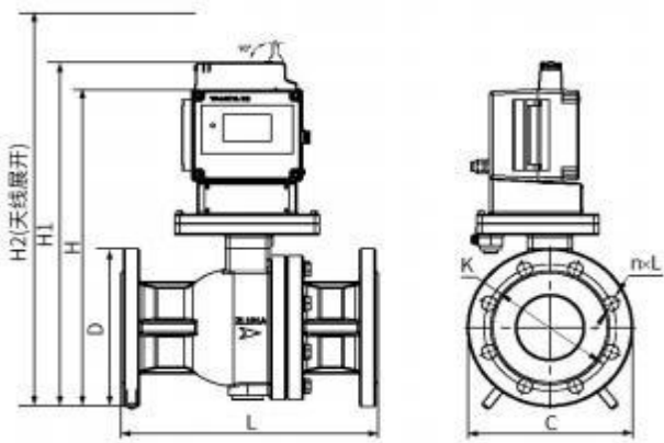
图 2-2 TCS-M 外型尺寸图
