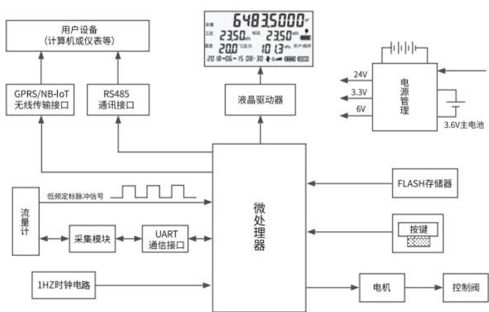
图 1 控制器原理框图
