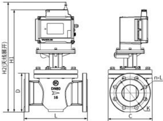
图 2-3 TCS-H 外型尺寸图
