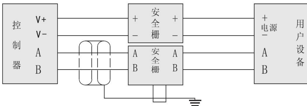
图 11 RS485 通信 (安全栅可选 GS8093)
