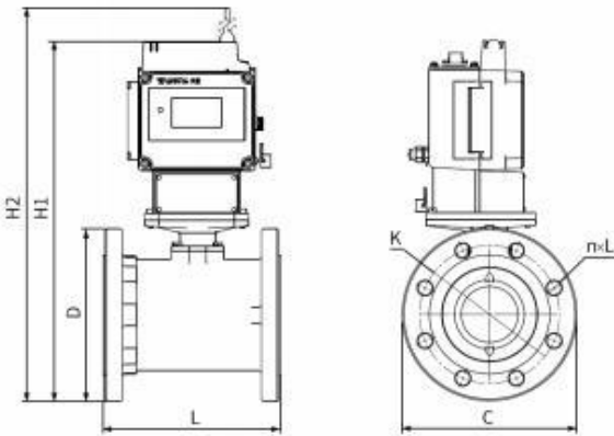
图 2-1 TCS-L 外型尺寸图
