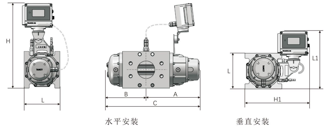
图5-3 TYLZ-G□-V
