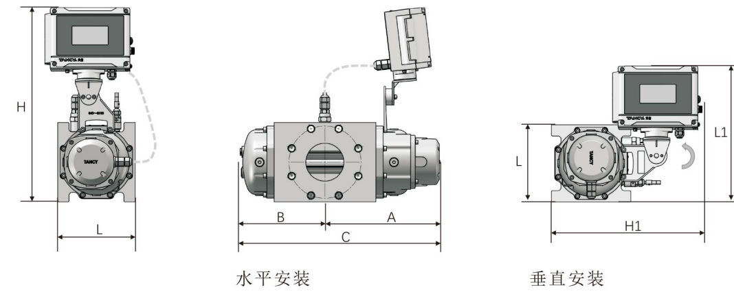
图5-1 TYLZ-G□
