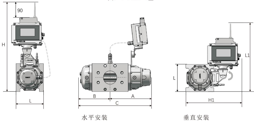
图5-1 TYLZ-G□
